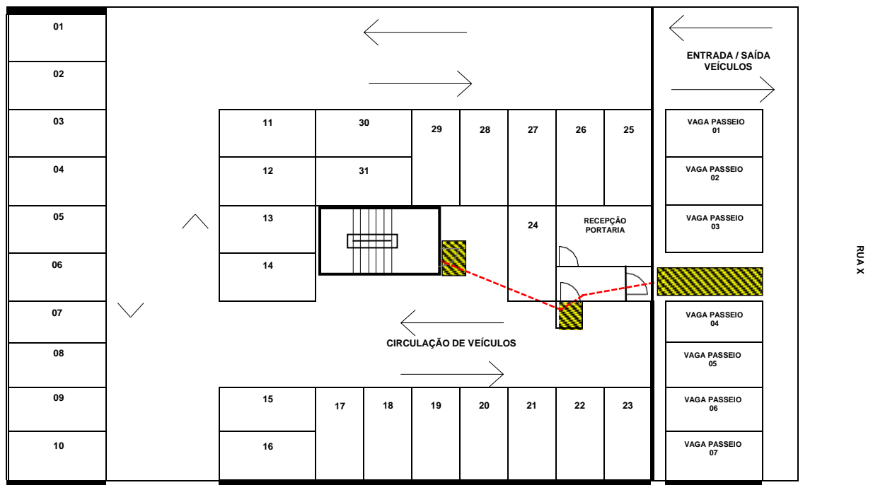
Figura B2 – Térreo garagem – Distância máxima a percorrer até saída da edificação (Área hachurada somente para fins explicativos)
