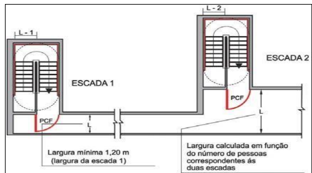
Figura 17 – Dimensionamento de corredores de descarga
