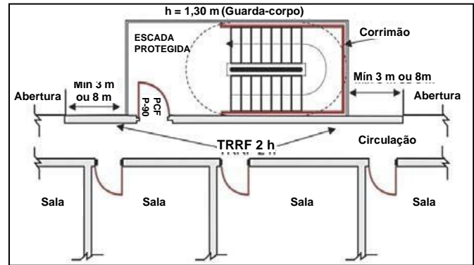
Figura 12 – Escada aberta externa
